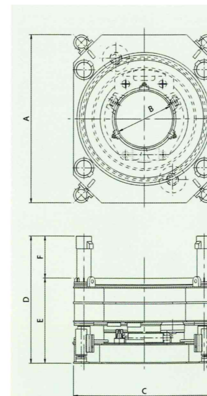
油圧式全回転スペースマシン仕様書
