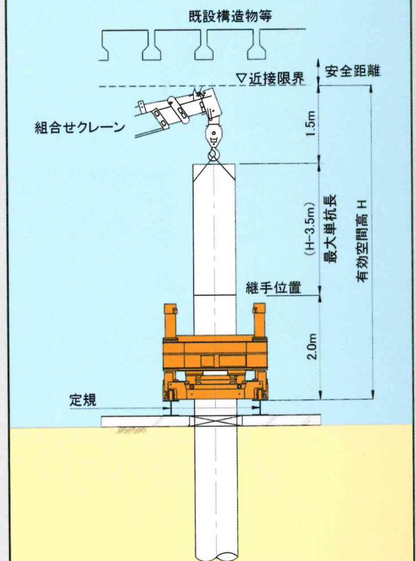
上空制限による杭施工限界長(標準)
